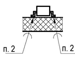
Установка VD1-VD4, VT1
