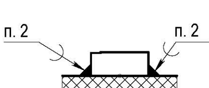
Установка C22-C24, C40
