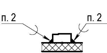
Установка C18
