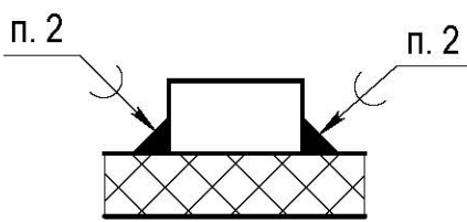
Установка C17, C21
