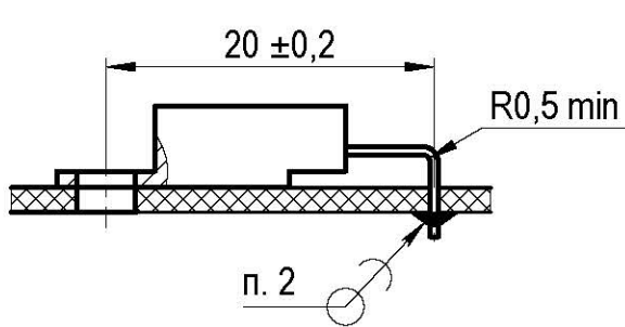
Установка DA1
