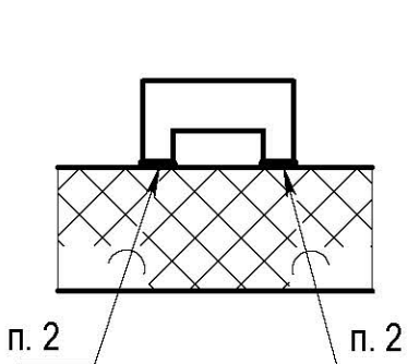
Установка L1
