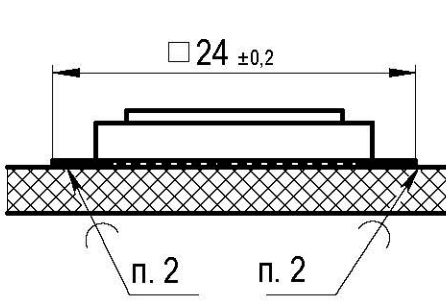
Установка DS2
