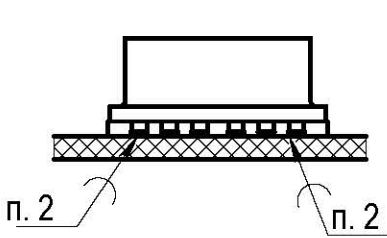
Установка T1-T4
