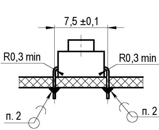
Установка SB1, SB2
