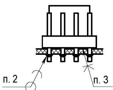
Установка XP16
