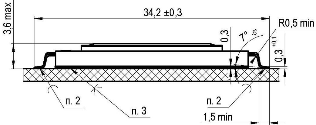
Установка D1, D2, DD1
