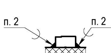
Установка C41, C74
