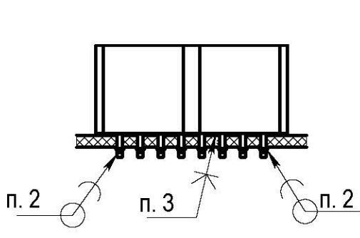
Установка XP5-XP7
