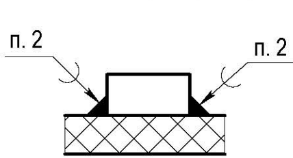
Установка C1-C9, C93, C94, C108
